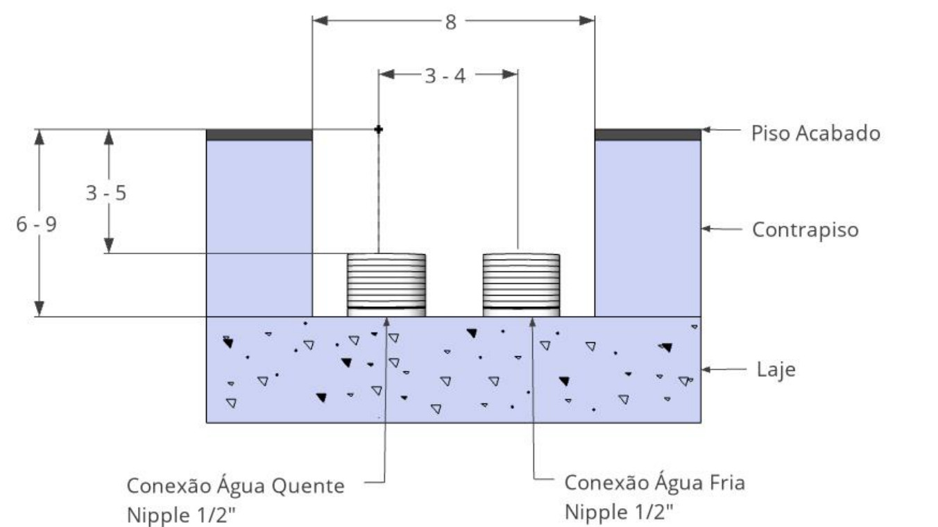
Detalhe - Instalação Hidráulica
